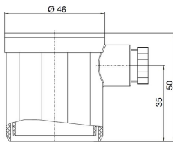
Beskyttelseshette med PG-forskruning Type 6371 (IP54) / 6372 (IP65)
