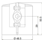
Beschermkap IP44 Type PC-PVS01-01
