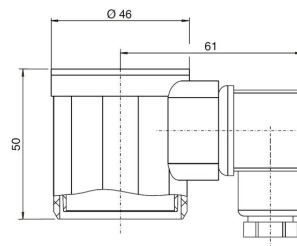
Beschermkap met apparaatcontactdoos IP65 Type 6379
