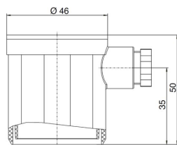
Beschermkap met PG-kabelwartel Type 6371 (IP54) / 6372 (IP65)
