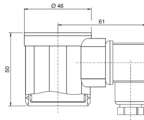
Beskyttelseskappe med apparatstikdåse IP65 Type 6379
