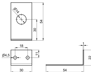
Γωνιακό στήριγμα Τύπος 6403
