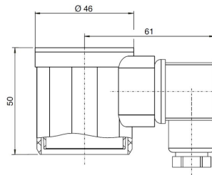
Προστατευτικό καπάκι με υποδοχή συσκευής IP65 Τύπος 6379
