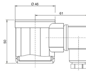
Beskyttelseshette med apparatkontakt IP65 Type 6379
