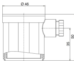
Beskyttelseshette med PG-forskrning Type 6371 (IP54) / 6372 (IP65)
