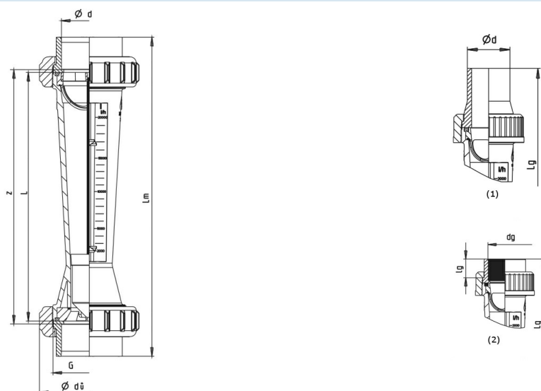
(1)...Racor con espiga para soldar, (2)...Racor con manguito roscado
