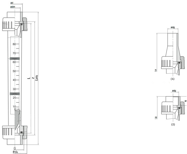
(1)...Racor con espiga para soldar, (2)...Racor con manguito roscado
