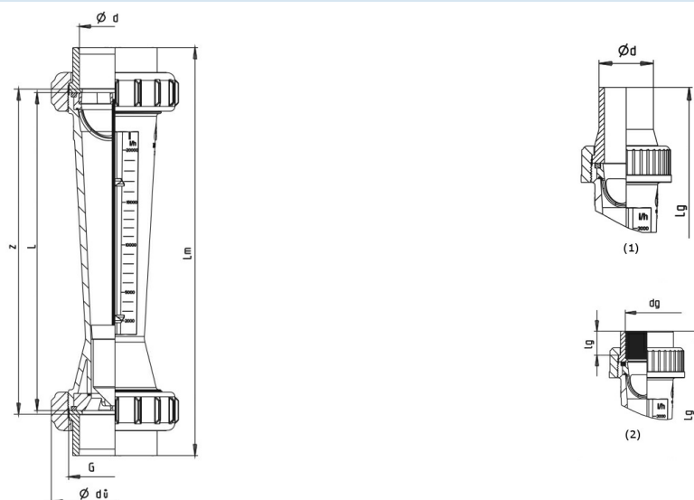
(1)...Raccord avec embout à souder, (2)...Raccord avec manchon fileté
