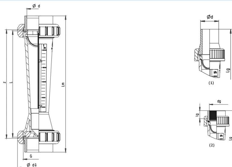
(1)...Raccordo con tronchetto a saldare, (2)...Raccordo con manicotto filettato
