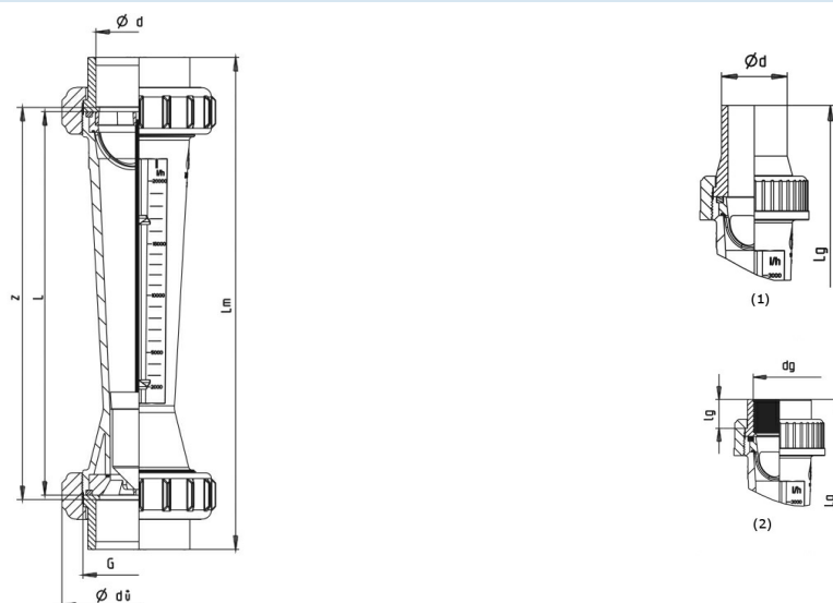
(1)...Skrukobling med sveisestuss, (2)...Skrukobling med gjengemuffe
