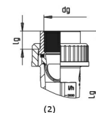
(1)...Skrukobling med sveisestuss, (2)...Skrukobling med gjengemuffe
