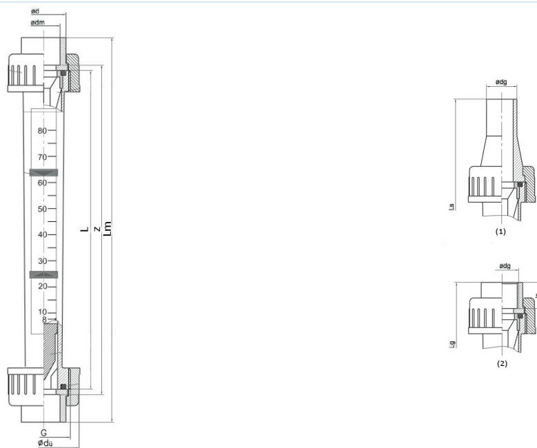
(1)...Racord cu stut de sudură, (2)...Racord cu manșon filetat
