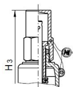
Testa tappo a tenuta di gas
