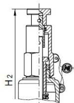
Cap de acționare etanș la gaz cu buton de aerisire
