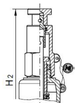
Huvud gastät med avluftningsknapp
