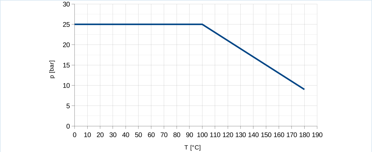
Diagramma pressione-temperatura:
