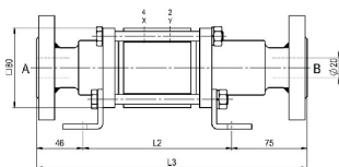
CVTE-20 Λειτουργία NC
