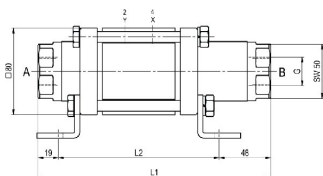
CVTE-20 Λειτουργία NC
