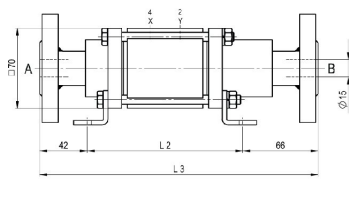
CVFE-15 Fonction NO
