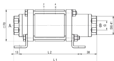
CVTE-15 Fonction NC
