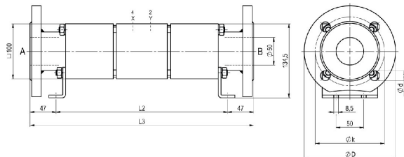
CVFV-50 Función NO
