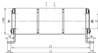
CVTV-50 Función NC
