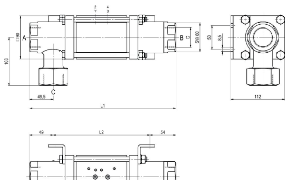
CVTE3-32 Λειτουργία NC
