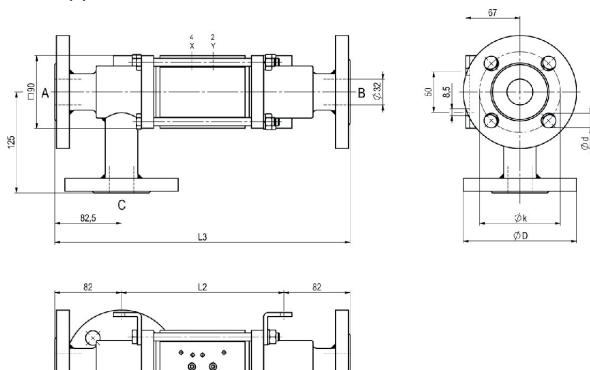
CVFE3-32 Λειτουργία NO
