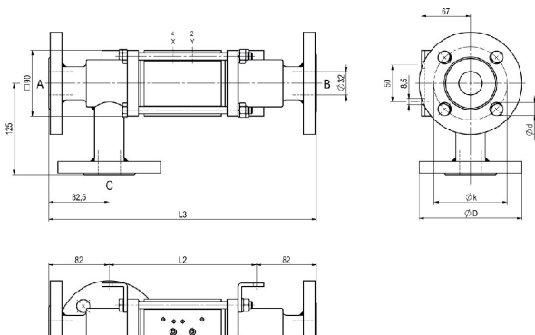
CVFE3-32 Toiminto NO
