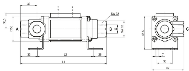
CVTE3-10 Funcție NC
