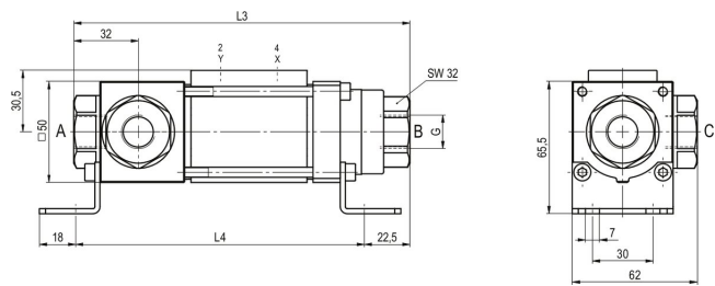
CVTE3-10 Funcție NC (> 63bar)
