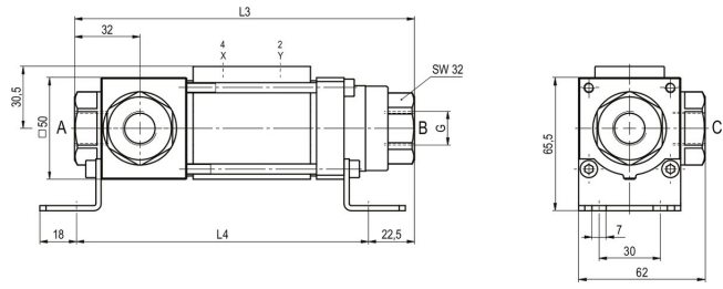
CVTE3-10 Funcție NO (> 63bar)
