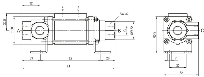
CVTE3-10 Funcție NO
