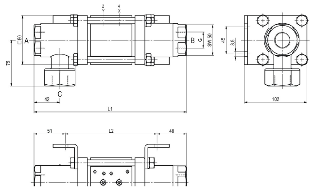
CVTE3-20 Funktion NC
