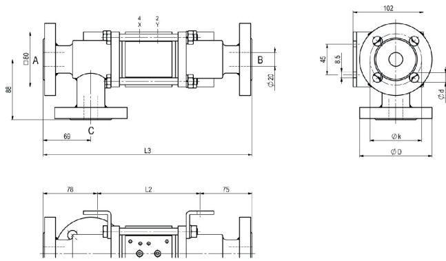
CVFE3-20 Funktion NO
