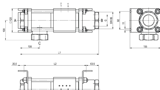
CVTE3-50 Λειτουργία NC
