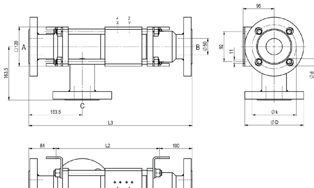
CVFE3-50 Λειτουργία NO
