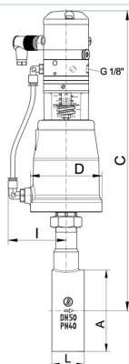
I/P-posisjonsregulator Type 8047
