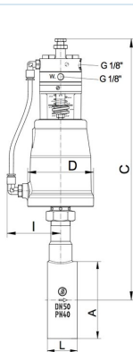
P/P-posisjonsregulator Type 8047
