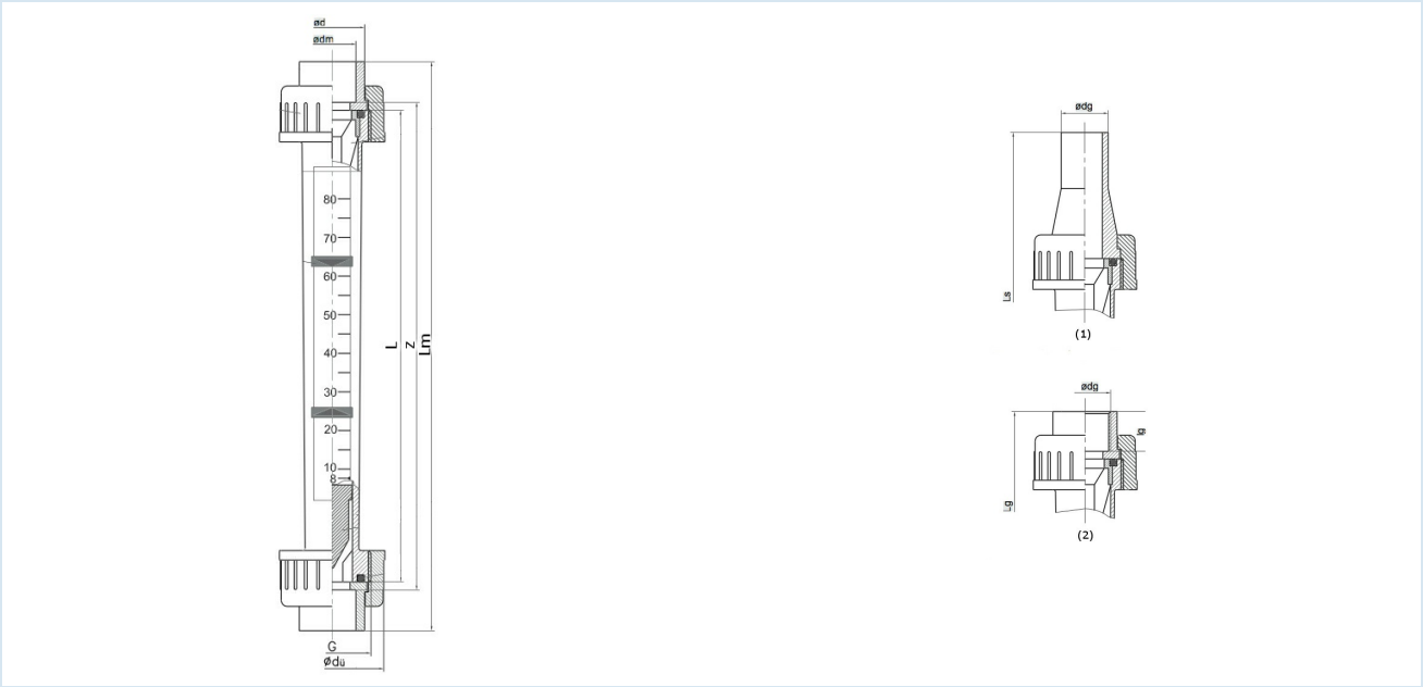
(1)...Racor con espiga para soldar, (2)...Racor con manguito roscado
