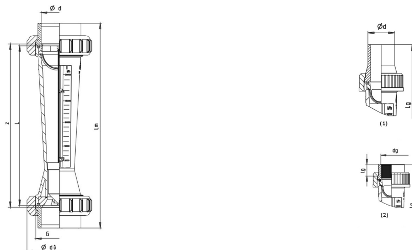
(1)...Hegeszthető csomos csavarzat, (2)...Menetes hüvelyes csatlakozó idom
