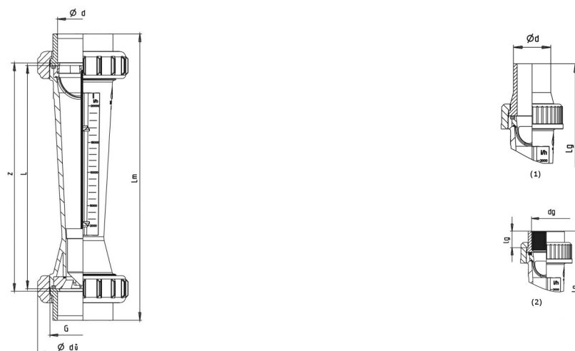
(1)...Raccordo con tronchetto a saldare, (2)...Raccordo con manicotto filettato
