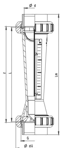
(1)...Skrukobling med sveistuss, (2)...Skrukobling med gjengemuffe
