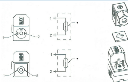
*Przyporządkowanie przyłączy Kontaktron (reed)
