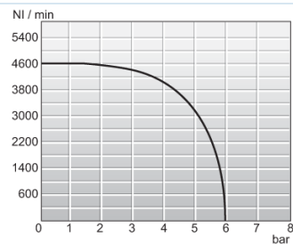
Διάγραμμα ροής 1/2"
