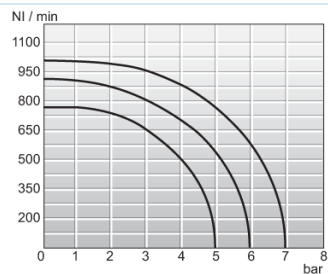
Διάγραμμα ροής 1/8"
