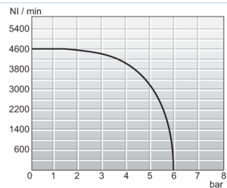
Átfolyási diagramm 1/2"
