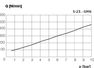
Przepływ
