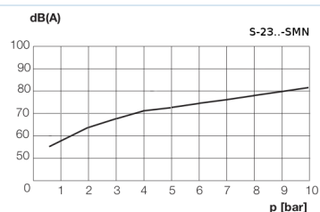
Poziom hałasu
