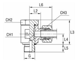
mit B3-Schneidring
