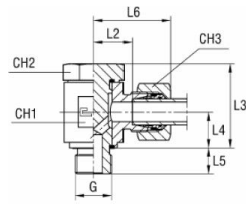
mit B4-Schneidring
