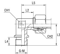
B3-leikkuurengasliitoksella
