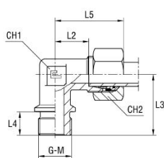
med B4-skjæring
