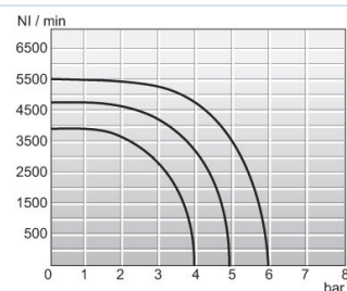
Virtauskaavio 1/2"
