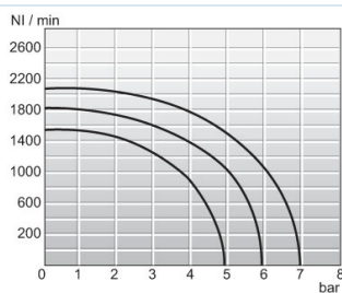
Virtauskaavio 1/4"
