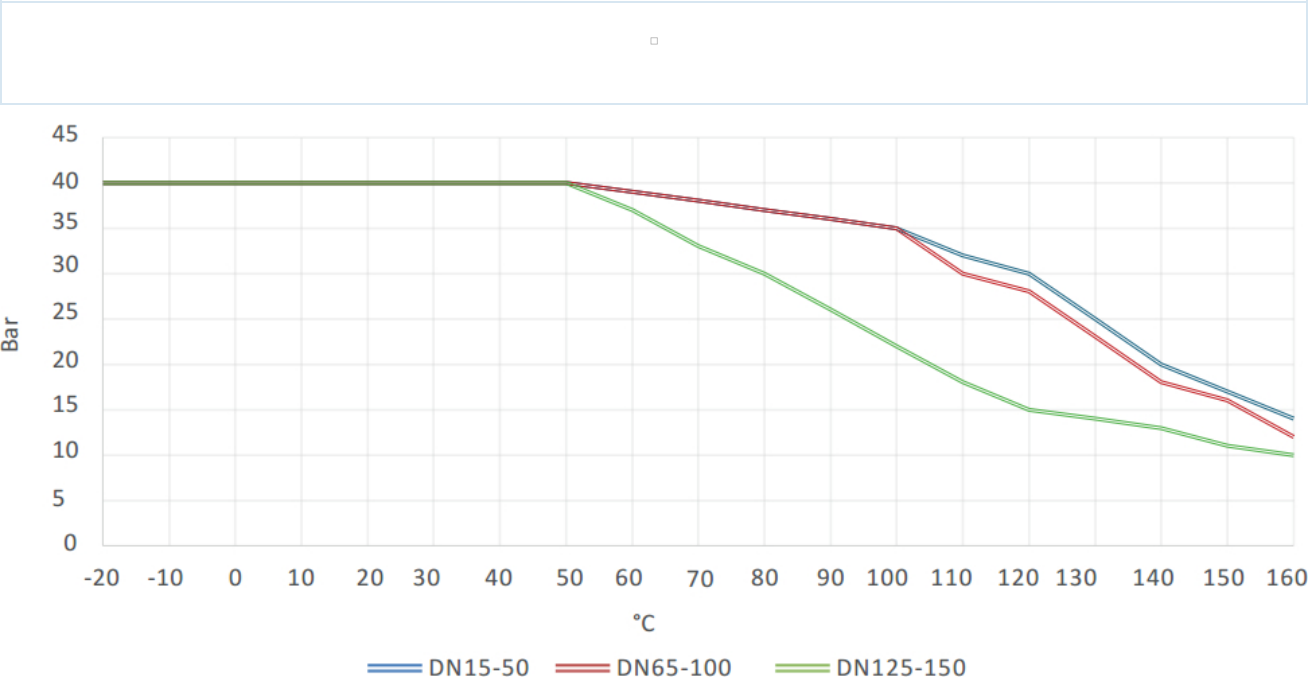
Diagramme pression-température
